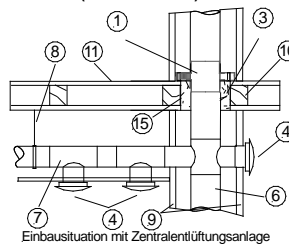
ST-ADW Einbau in, auf u. unter Geschossdecke gemäß Anlage 4 aus Holz (Holzbalkendecke) F 30 - F 90 / variabler Einbau der ST-ADW pro Strang möglich
