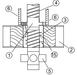
Einbau auf der Geschossdecke aus Holz, Holzbalkendecke F 30-B - F 90-B
