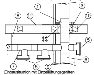
ST-ADW Einbau in, auf u. unter Geschossdecke gemäß Anlage 4 aus Holz (Holzbalkendecke) F 30 - F 90 / variabler Einbau der ST-ADW pro Strang möglich
