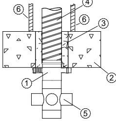
Einbau in der Geschossdecke aus Beton oder Porenbeton F 30 - F90
