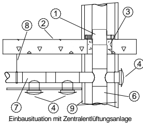
ST-ADW Einbau in, auf u. unter Geschossdecke gemäß Anlage 3 aus Beton F 30 - F 90 / variabler Einbau der ST-ADW pro Strang möglich
