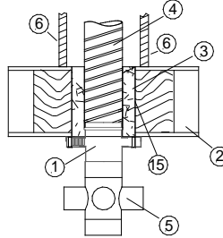
Einbau in der Geschossdecke aus Holz, Holzbalkendecke F 30-B - F 90-B
