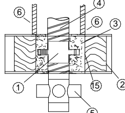
Einbau in der Geschossdecke aus Holz, Holzbalkendecke F 30-B - F 90-B
